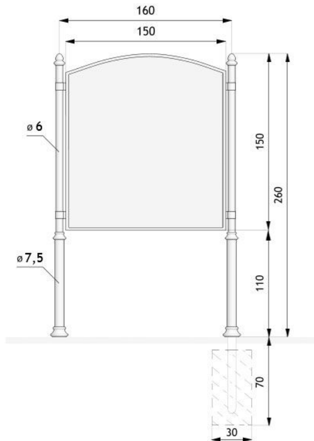
wymiary podane w [cm]
